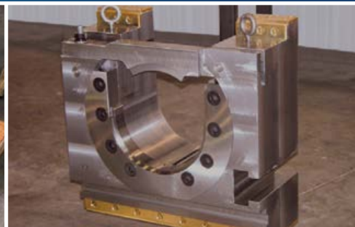
New Die Shuffle
